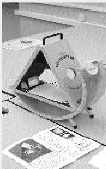
Telescopi solar.
