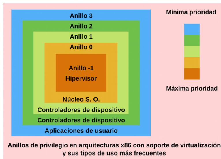
Figura 1: Anillos de privilegio en x86
