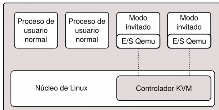
Figura 3: Arquitectura de KVM
