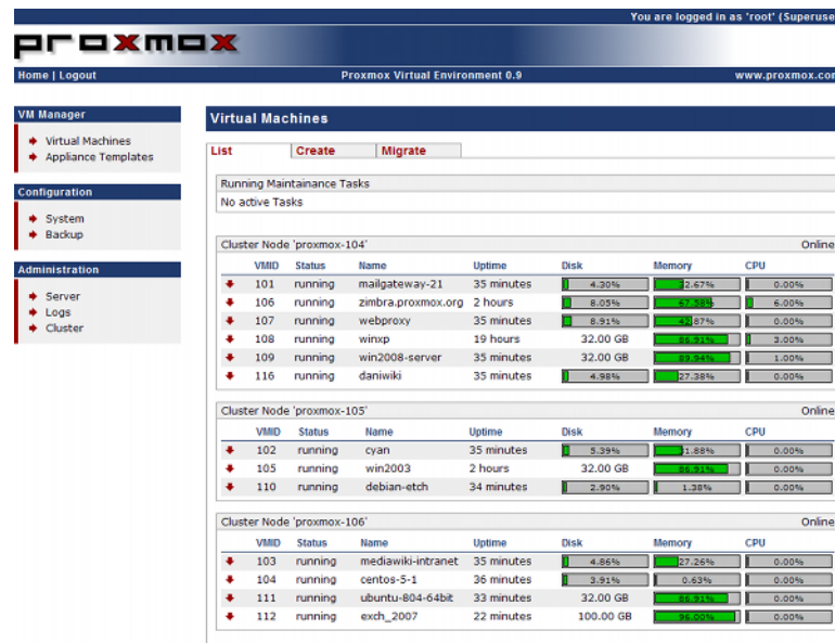
Figura 4: Listado de máquinas virtuales en un cluster ProxmoxVE
