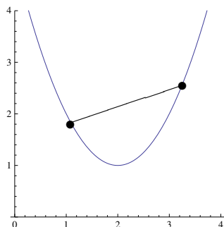
Función convexa
