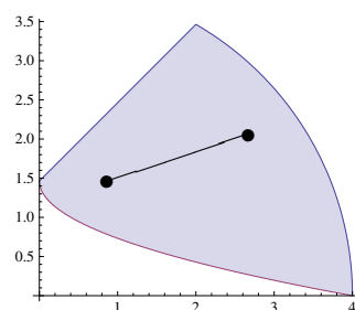
Conjunto convexo
