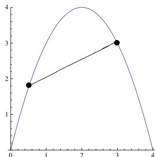
Función cóncava
