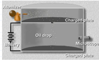
Experimento de Millikan
