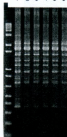
Fig. 4 RAPD de diferentes aislados de O. oeni . Carreras 1 y 14: 1 KB plus ladder (Invitrogen). Carrera 2: Cepa control inoculada. Carreras 3-8: aislados de O. oeni de vino.
