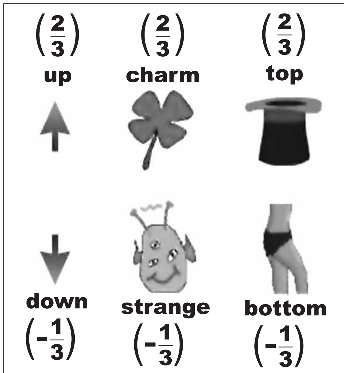
Els sis quarks coneguts, anomenats en anglés up, down, strange, charm, beauty i top. Els nombres fraccionaris fan referència a la seua càrrega elèctrica en unitats de la càrrega de l'electró.
