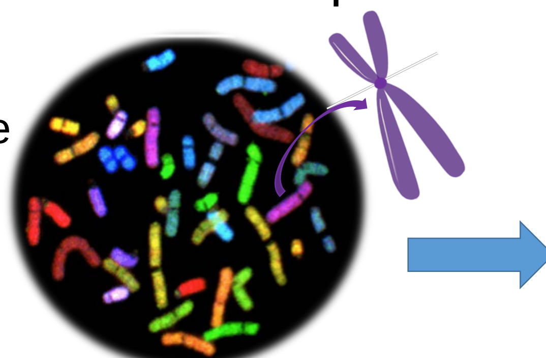
Cariotip humà
