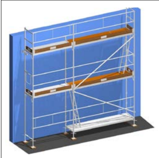
Figura 7. Ejemplo de andamio con las protecciones colectivas instaladas en los niveles de trabajo.
