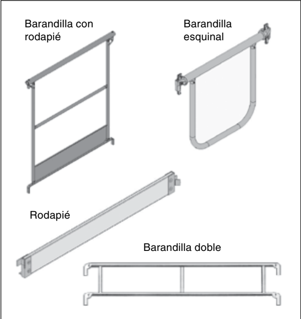
Figura 6. Protecciones colectivas perimetrales. Elementos.
