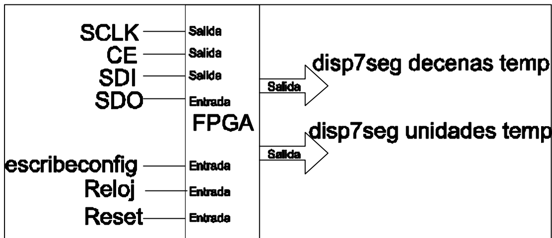
Figura que muestra las líneas externas (así como si son de Entrada o Salida) de la FPGA a diseñar.
