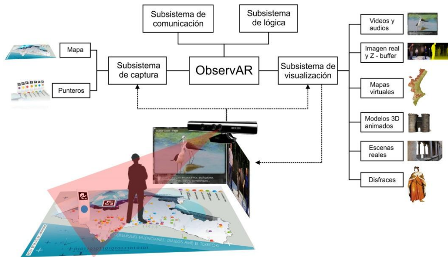
Fig. 2. Diagrama de componentes del sistema ObservAR
