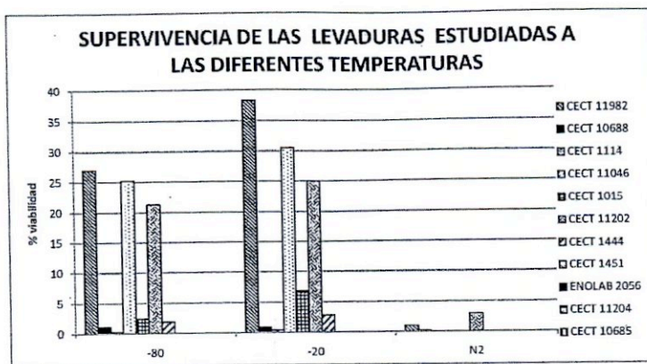
Fig1: Supervivencia media, expresada en %, de las levaduras estudiadas en relación a las distintas temperaturas de congelación ensayadas. En las cepas CECT 1451, 2056, 11204 y 10685 no se aprecian en la figura por exhibir porcentajes de supervivencia muy reducidos.
