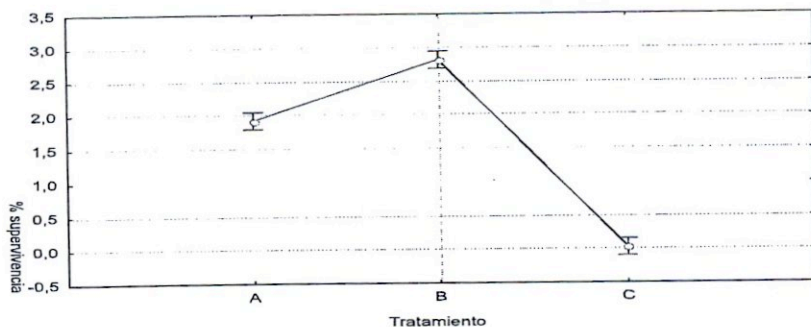
Fig.2. Resultados obtenidos con la cepa CECT 1444 frente a las distintas temperaturas de congelación previa a la liofilización. (A: -80°C, B: -20°C, C: nitrógeno líquido)
