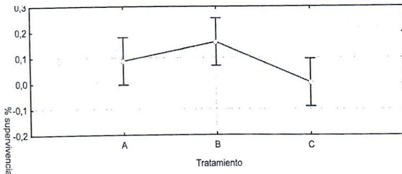
Fig3: Gráfica en la cual mostramos el comportamiento de la cepa CECT 1114 frente a las distintas temperaturas de congelación previa a la liofilización. (A: -80°C, B: -20°C, C: nitrógeno líquido)
